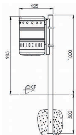
Pfostenbefestigung
