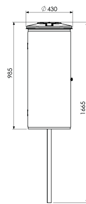
Vorderansicht 8059-11 zum Einbetonieren
