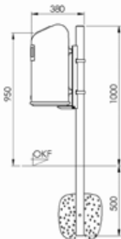
Pfostenbefestigung
