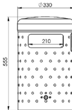
Frontansicht
