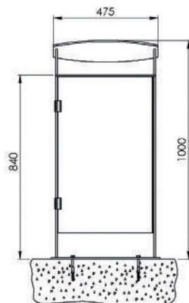
Frontansicht Ausführung zum Aufschrauben
