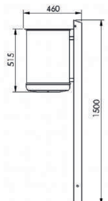
7039-15 Seitenansicht
