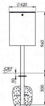
Frontansicht
