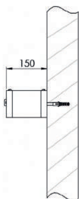
Modell 7068-00 Wandbefestigung
