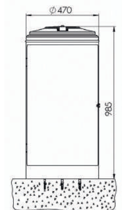
Montage auf Betonfundament
