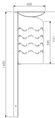
Seitenansicht zum Einbetonieren
