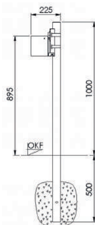
Pfostenbefestigung
