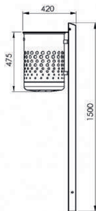
7038-00 Seitenansicht
