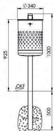
7038-00 Frontansicht
