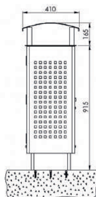
Frontansicht
