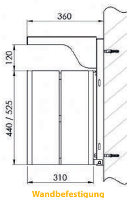
Wandbefestigung
