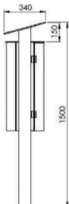
Seitenansicht
