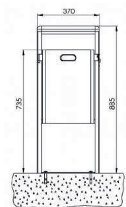
Frontansicht zum Aufschrauben 7083-30
