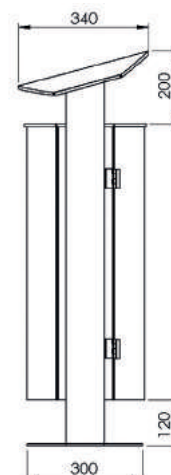
Seitenansicht
