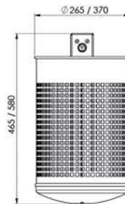
Frontansicht
