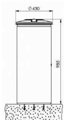
Vorderansicht 8059-00 zum Aufschrauben
