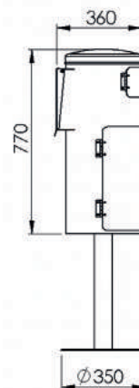
7077-01 Seitenansicht
