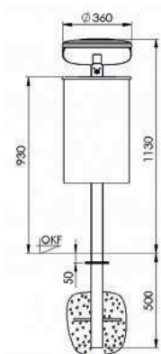
Frontansicht
