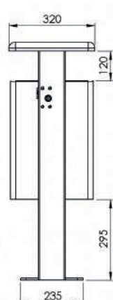
Seitenansicht zum Aufschrauben 7083-30
