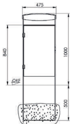
Frontansicht Ausführung zum Einbetonieren
