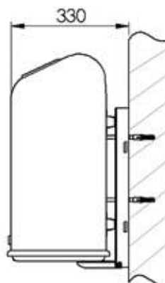
Wandbefestigung
