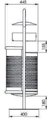
7031-62 Seitenansicht
