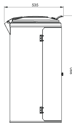
Seitenansicht
