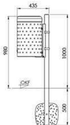
Pfostenbefestigung
