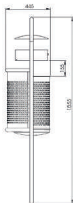
7031-52 Seitenansicht
