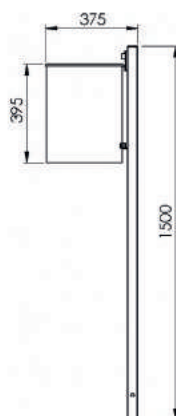
Seitenansicht
