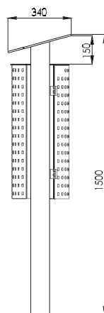
Seitenansicht
