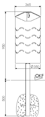
Frontansicht zum Einbetonieren
