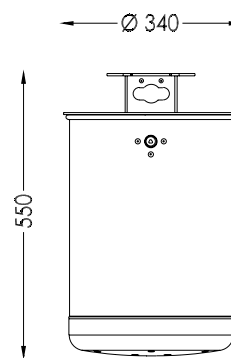
Frontansicht
