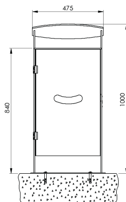
Frontansicht Ausführung zum Aufschrauben
