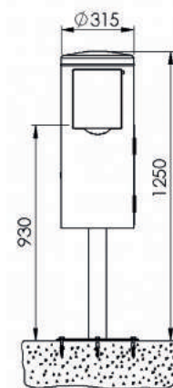
7077-01 Frontansicht zum Aufschrauben
