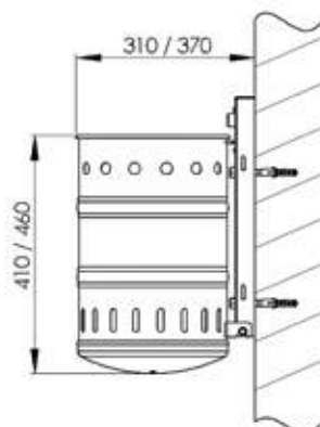
Wandbefestigung
