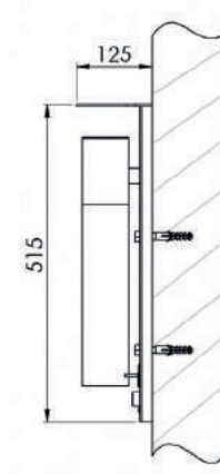
Modell 7061-01 Wandbefestigung
