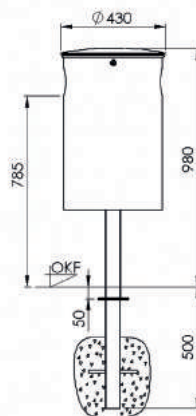
Frontansicht
