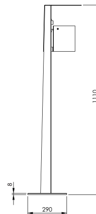
7070 S-00 Seitenansicht
