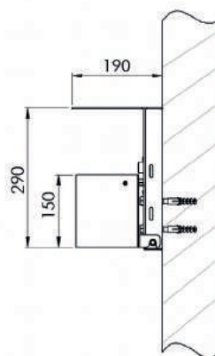
Wandbefestigung
