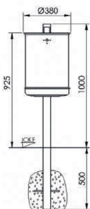
Frontansicht
