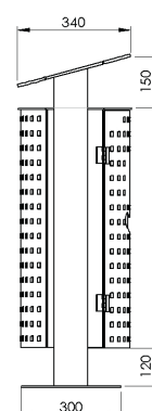
Seitenansicht
