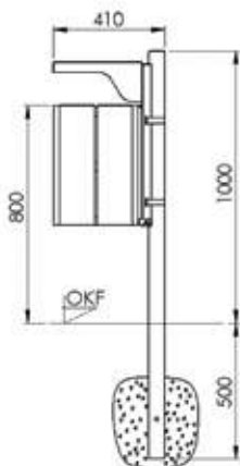
Pfostenbefestigung
