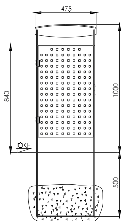
Frontansicht Ausführung zum Einbetonieren
