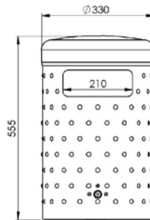
Frontansicht
