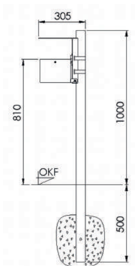
Pfostenbefestigung
