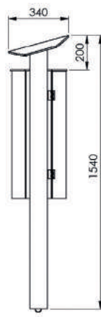
Seitenansicht
