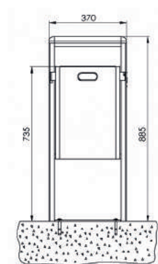
Frontansicht zum Aufschrauben 7083-60
