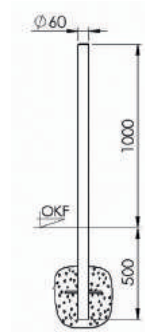
Abb.: Montageempfehlung Pfosten zum Einbetonieren
