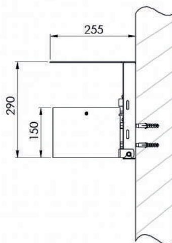
Wandbefestigung
