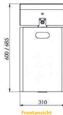
Frontansicht
