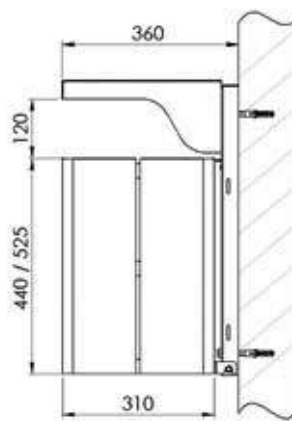
Wandbefestigung
