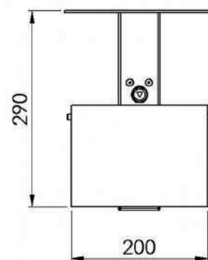
Frontansicht
