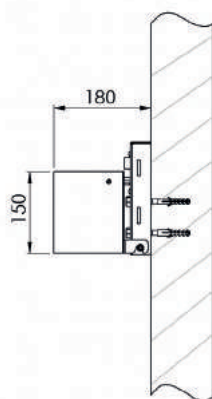
Wandbefestigung
