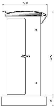
Seitenansicht 8059-10 zum Aufschrauben mit optionalem Betonsockel 7050-03
