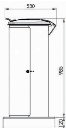
Seitenansicht 8059-00 zum Aufschrauben mit optionalem Betonsockel 7050-03
