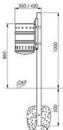
Pfostenbefestigung
