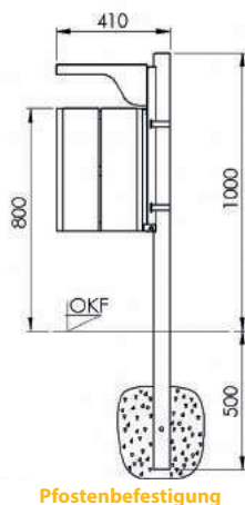
Pfostenbefestigung
