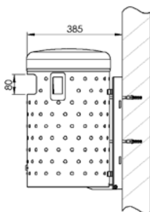
Wandbefestigung
