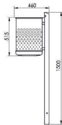
7039-00 Seitenansicht
