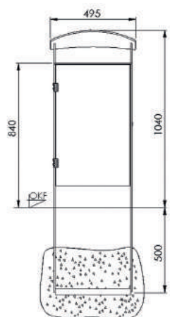
Frontansicht Ausführung zum Einbetonieren
