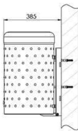
Wandbefestigung
