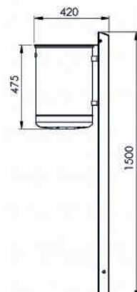
7038-15 Seitenansicht
