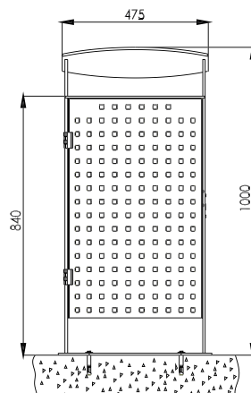
Frontansicht Ausführung zum Aufschrauben
