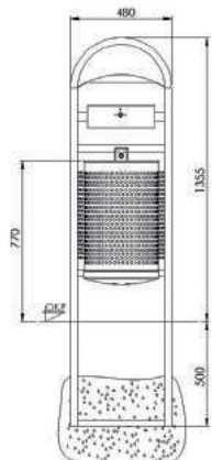
7031-52 Frontansicht Ausführung zum Einbetonieren
