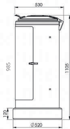
Montage auf optionalem Betonsockel 7050-03
