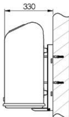
Wandbefestigung
