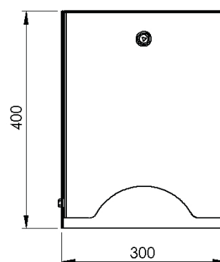
Frontansicht
