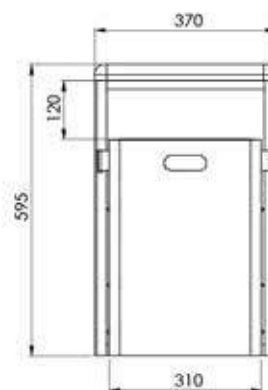
Frontansicht
