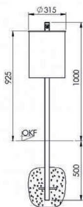
Frontansicht
