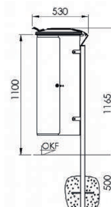
Seitenansicht 8059-01 zum Einbetonieren
