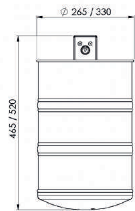
Frontansicht
