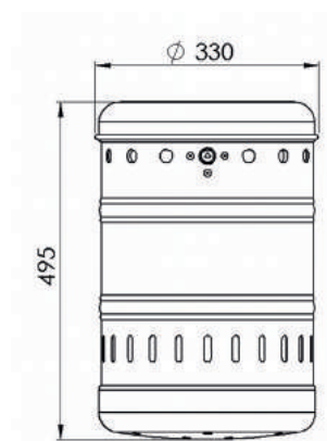
Frontansicht
