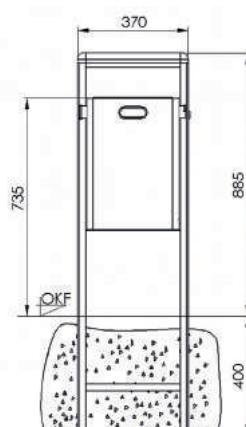
Frontansicht zum Einbetonieren 7083-40
