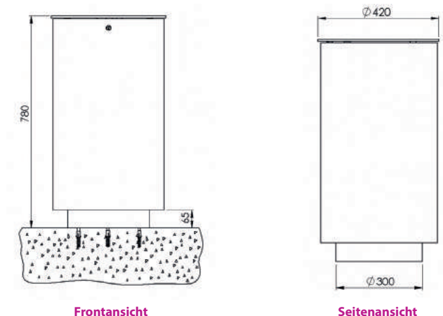
Frontansicht
