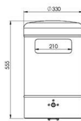
Frontansicht
