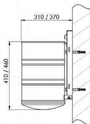
Wandbefestigung
