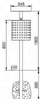
Frontansicht Ausführung zum Einbetonieren
