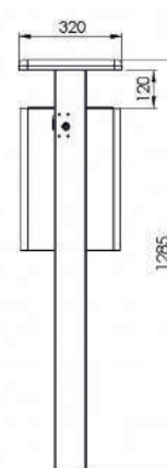
Seitenansicht zum Einbetonieren 7083-40
