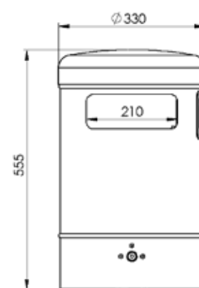
Frontansicht
