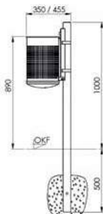
Pfostenbefestigung
