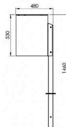
Seitenansicht
