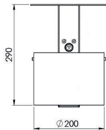
Frontansicht
