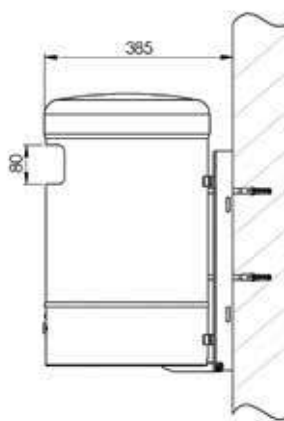
Wandbefestigung
