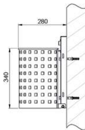
Wandbefestigung
