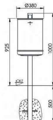
7039-15 Frontansicht
