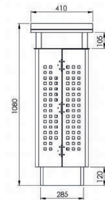
Seitenansicht
