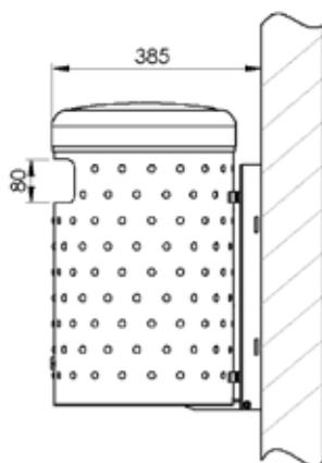
Wandbefestigung
