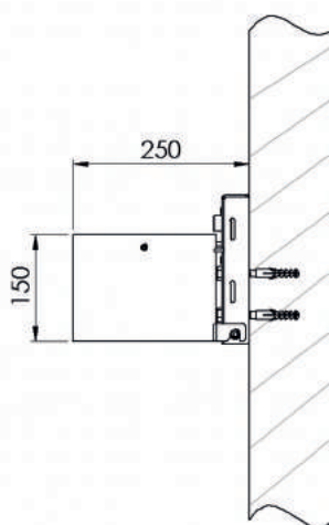
Wandbefestigung
