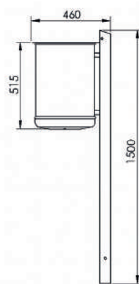
Seitenansicht
