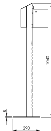
7067 S-01 Seitenansicht
