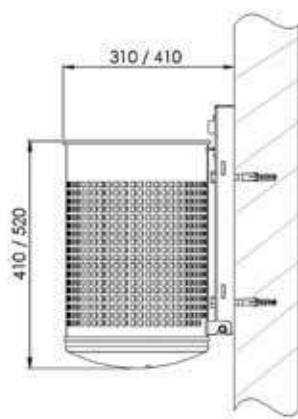
Wandbefestigung
