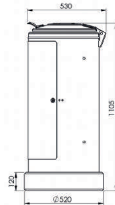
Montage auf optionalem Betonsockel 7050-03
