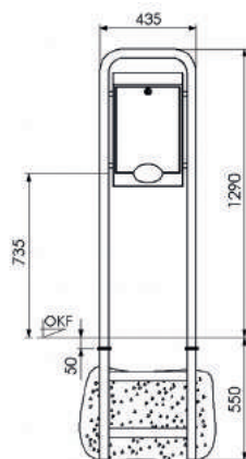
Frontansicht
