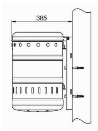
Wandbefestigung
