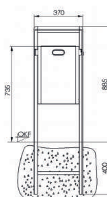
Frontansicht zum Einbetonieren 7083-70
