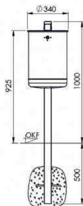
7038-15 Frontansicht
