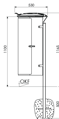
Seitenansicht 8059-11 zum Einbetonieren
