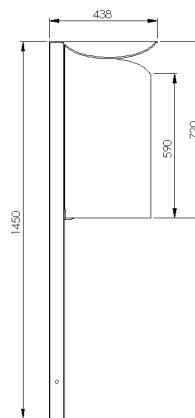
Seitenansicht zum Einbetonieren
