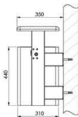
Wandbefestigung
