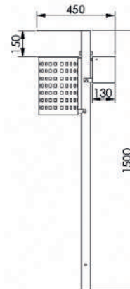
Seitenansicht
