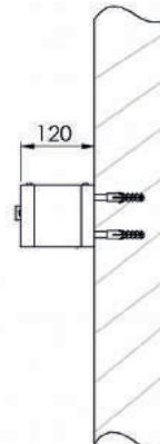
Modell 7068-10 Wandbefestigung
