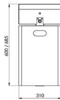
Frontansicht
