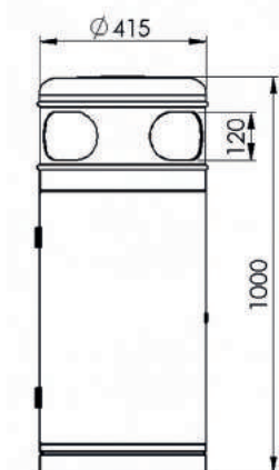
Frontansicht
