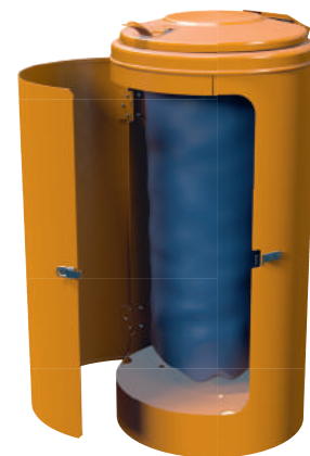
Abb.: 8045-20 in RAL 2000 (Sonderfarbe)
