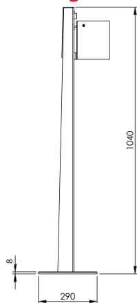
7067 S-00 Seitenansicht
