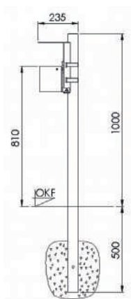
Pfostenbefestigung
