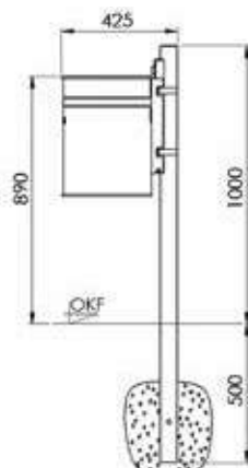
Pfostenbefestigung
