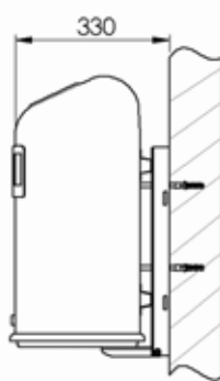
Wandbefestigung
