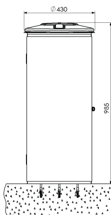
Vorderansicht 8059-10 zum Aufschrauben
