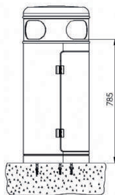
Seitenansicht
