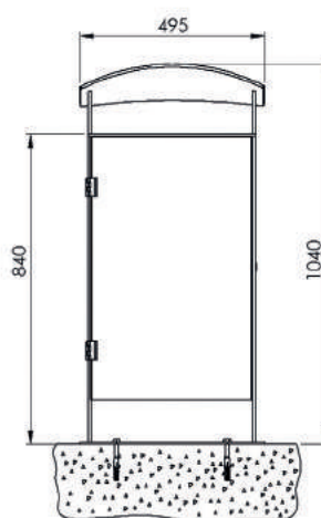
Frontansicht Ausführung zum Aufschrauben
