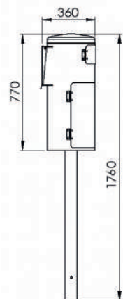
7077-00 Seitenansicht
