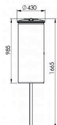
Vorderansicht 8059-01 zum Einbetonieren
