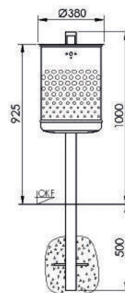
7039-00 Frontansicht
