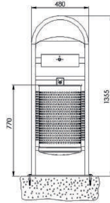
7031-62 Frontansicht Ausführung zum Aufschrauben
