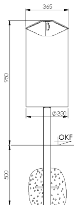
Frontansicht zum Einbetonieren
