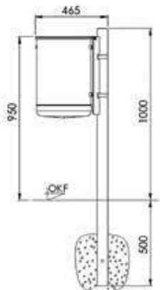
Pfostenbefestigung
