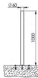
Abb.: Montageempfehlung Pfosten zum Aufschrauben
